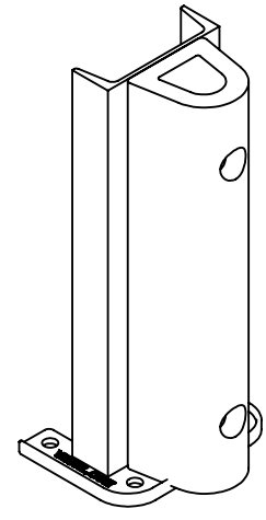
3-D VIEW SCALE: 1:8
