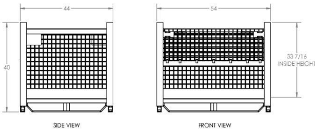
DIMENSIONS
